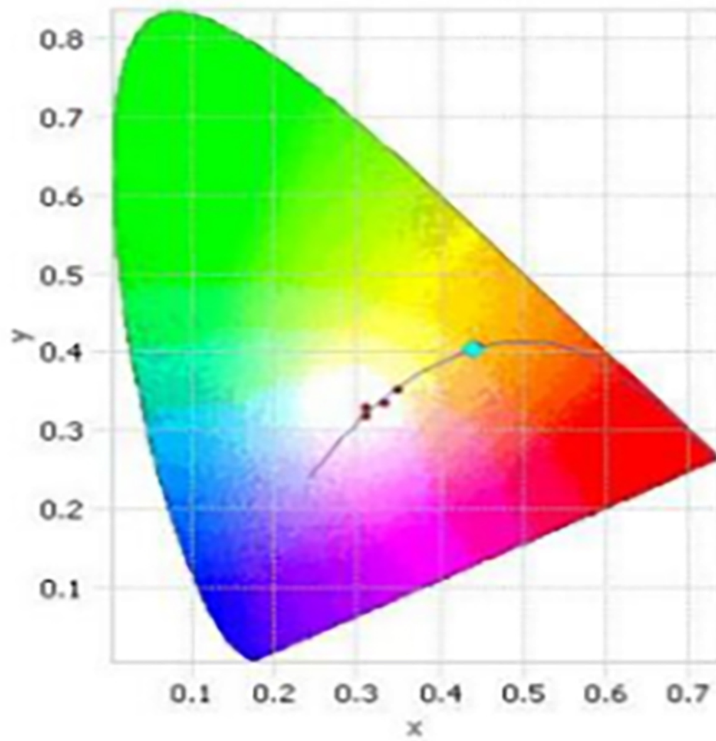
CIE 1931, 2 Degree
